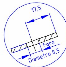
PIEDE SOSTEGNO SCALA 1:5
