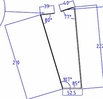
PIEDE SOSTEGNO SCALA 1:5
